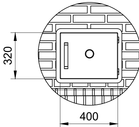
A (1:16) Puerta del horno
